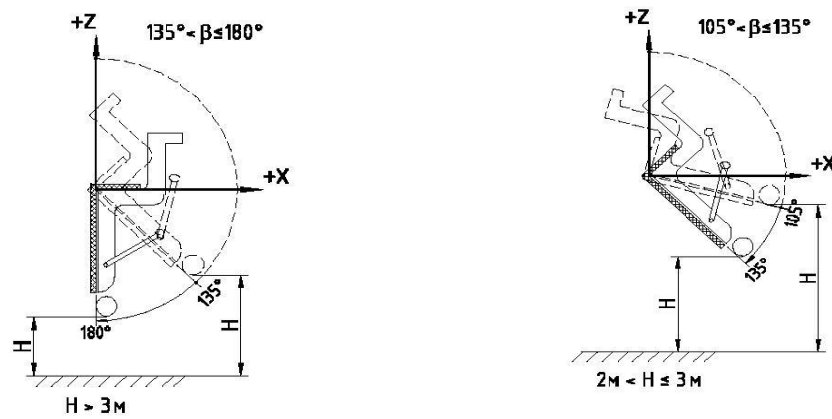
Рисунок 2. Наклон пассажирских кресел назад
