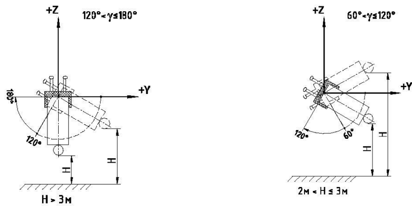
Рисунок 3. Наклон пассажирских кресел набок
