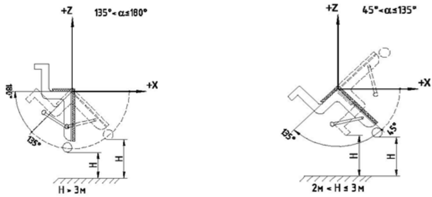
Рисунок 1. Наклон пассажирских кресел вперед
