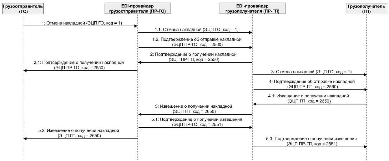
Рисунок 3.12 - Диаграмма последовательности отмены накладной грузоотправителем (два EDI-провайдера)
